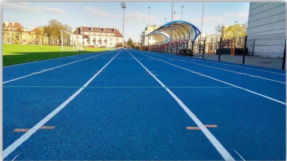
Przebudowa stadionu miejskiego przy ul. Świętokrzyskiej w Sierpcu – budowa z przebudową bieżni lekkoatletycznej oraz urządzeniami i infrastrukturą towarzyszącą.
